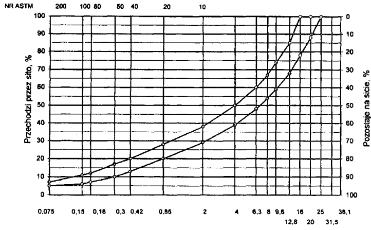
Wymiary oczek sit kwadratowych, mm
