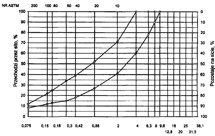
Wymiary oczek sit kwadratowych, mm
